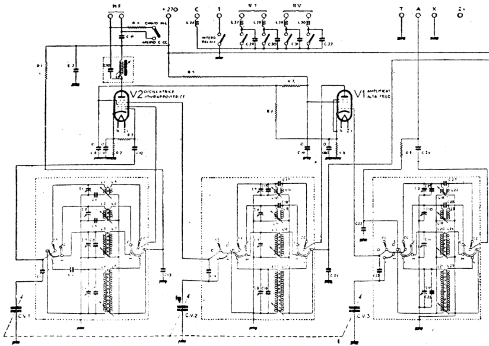
PHONOLA (S. A. FIMI). — Mod. « 910 » (Telesinto).
